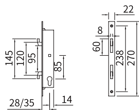
Hook mortise
